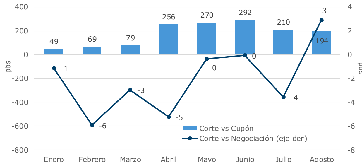
Diferencial tasas de corte subastas TES vs Tasas Negociación TES y Cupón TES
