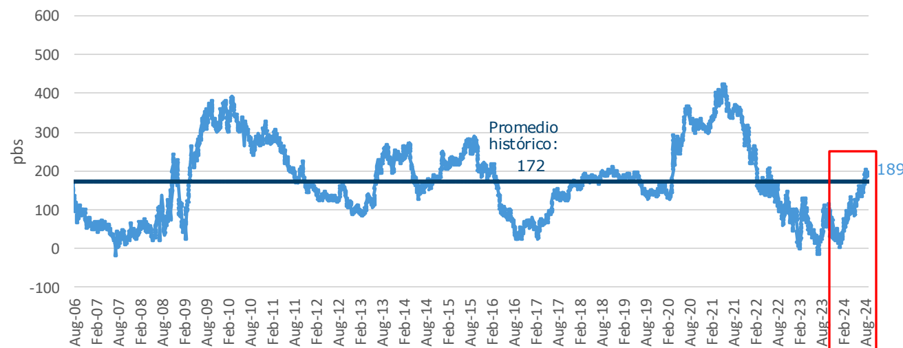
Pendiente Curva Cero Cupón TES entre 2/10 años
